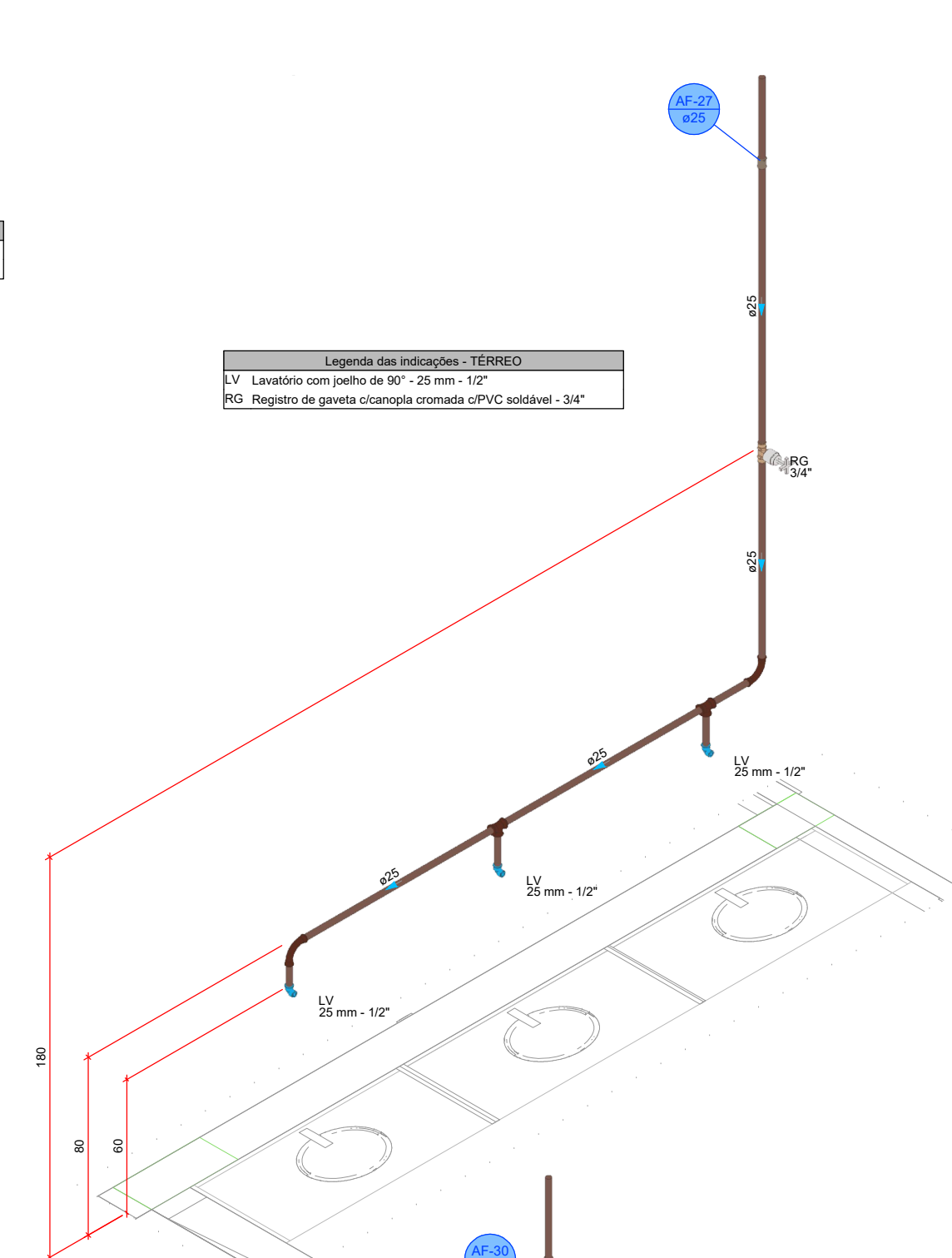
DETALHE HID-25 1:20
