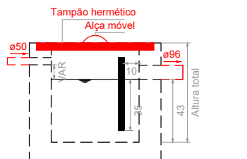
Caixa de gordura - TERREO Corte 1 - ESC. 1:25
