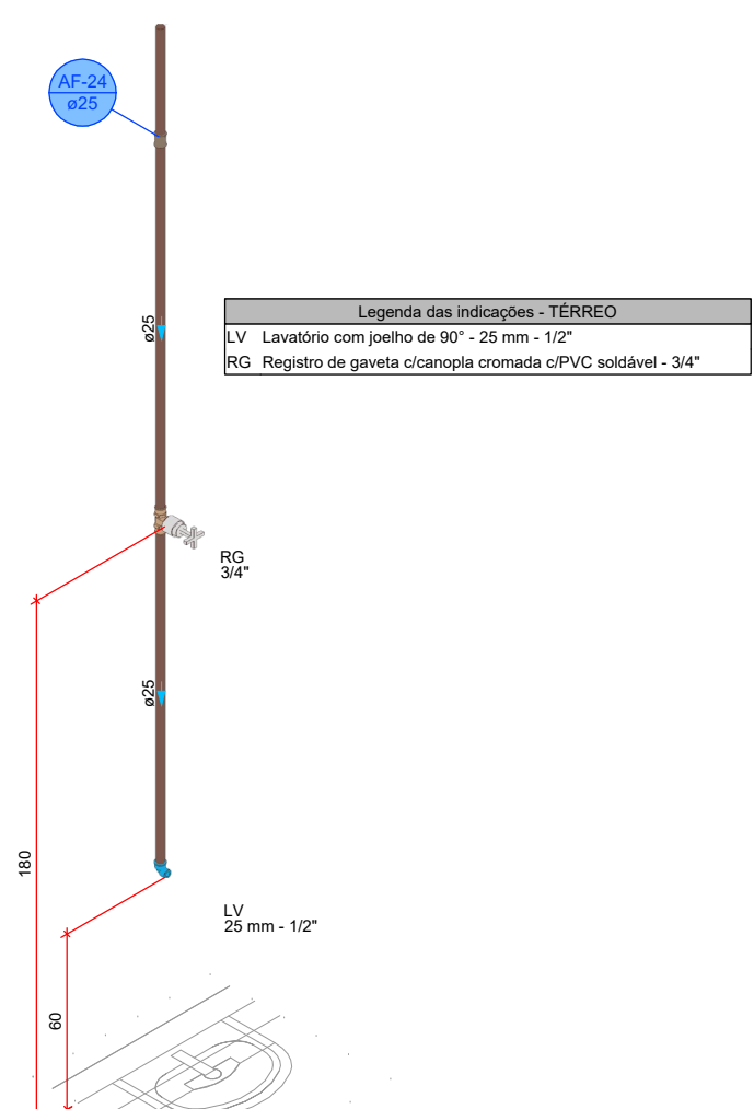
DETALHE HID-23 1:20
