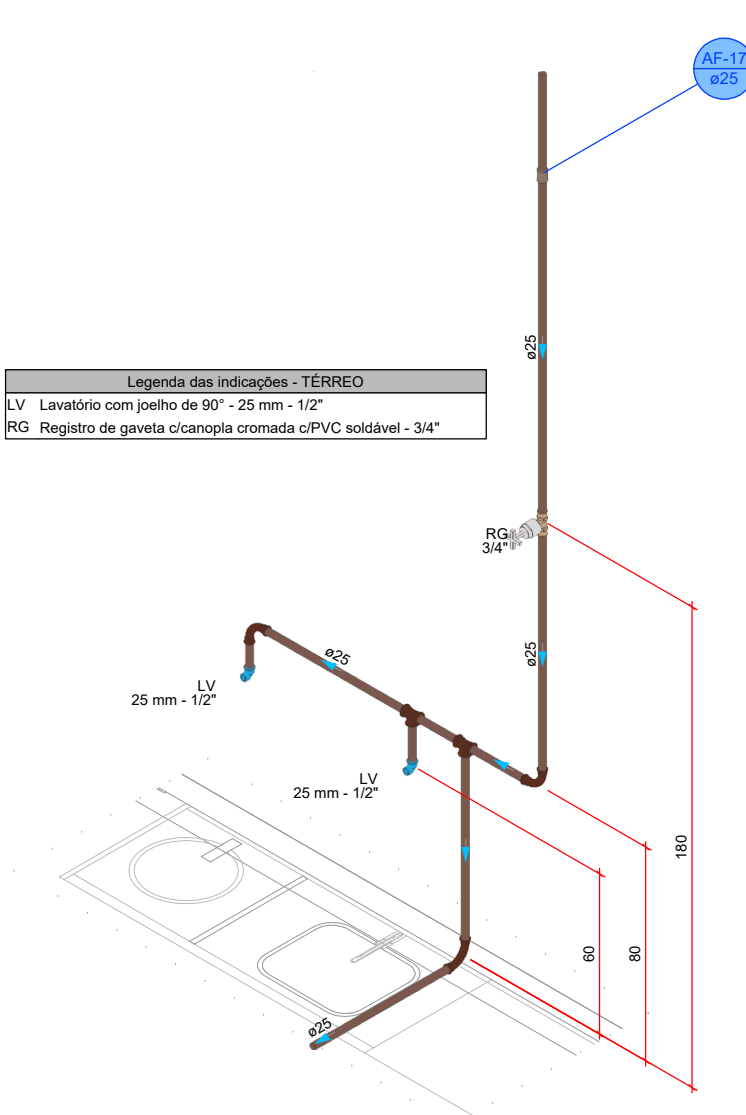
DETALHE HID-16 1:20
