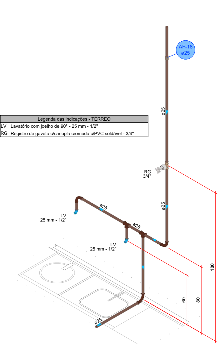
DETALHE HID-17 1:20
