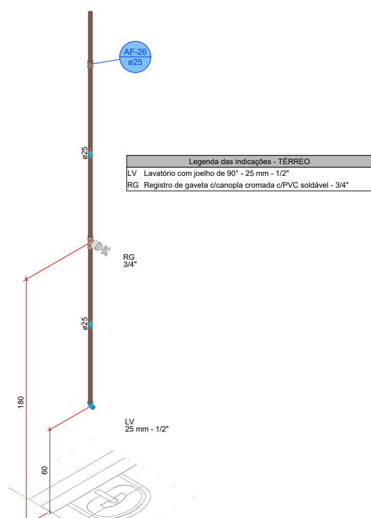
DETALHE HID-22 1:20
