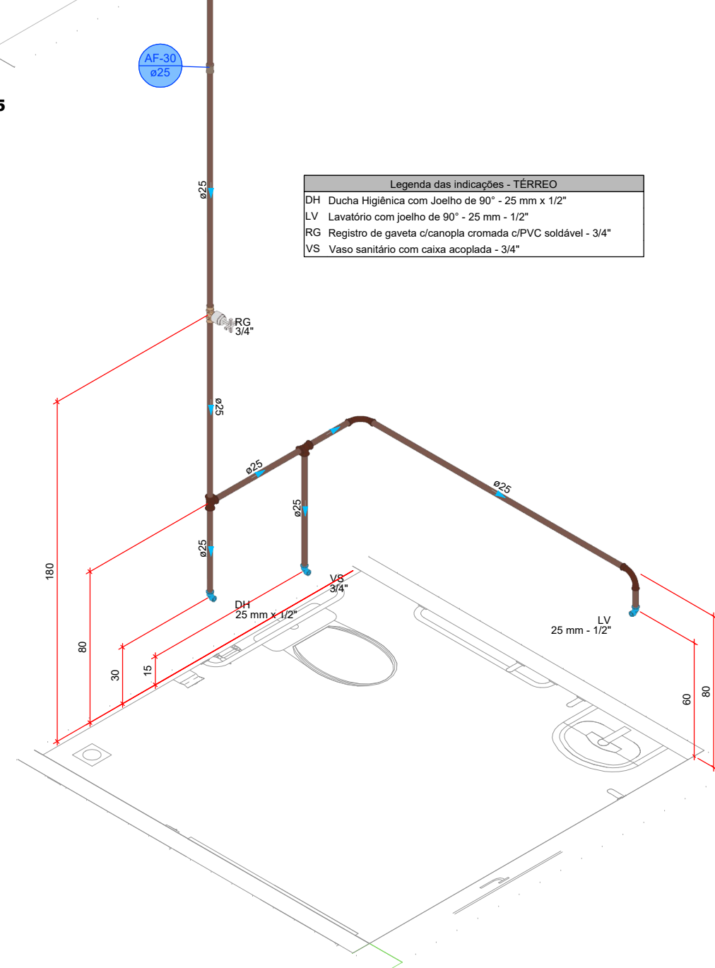
DETALHE HID-30 1:20
