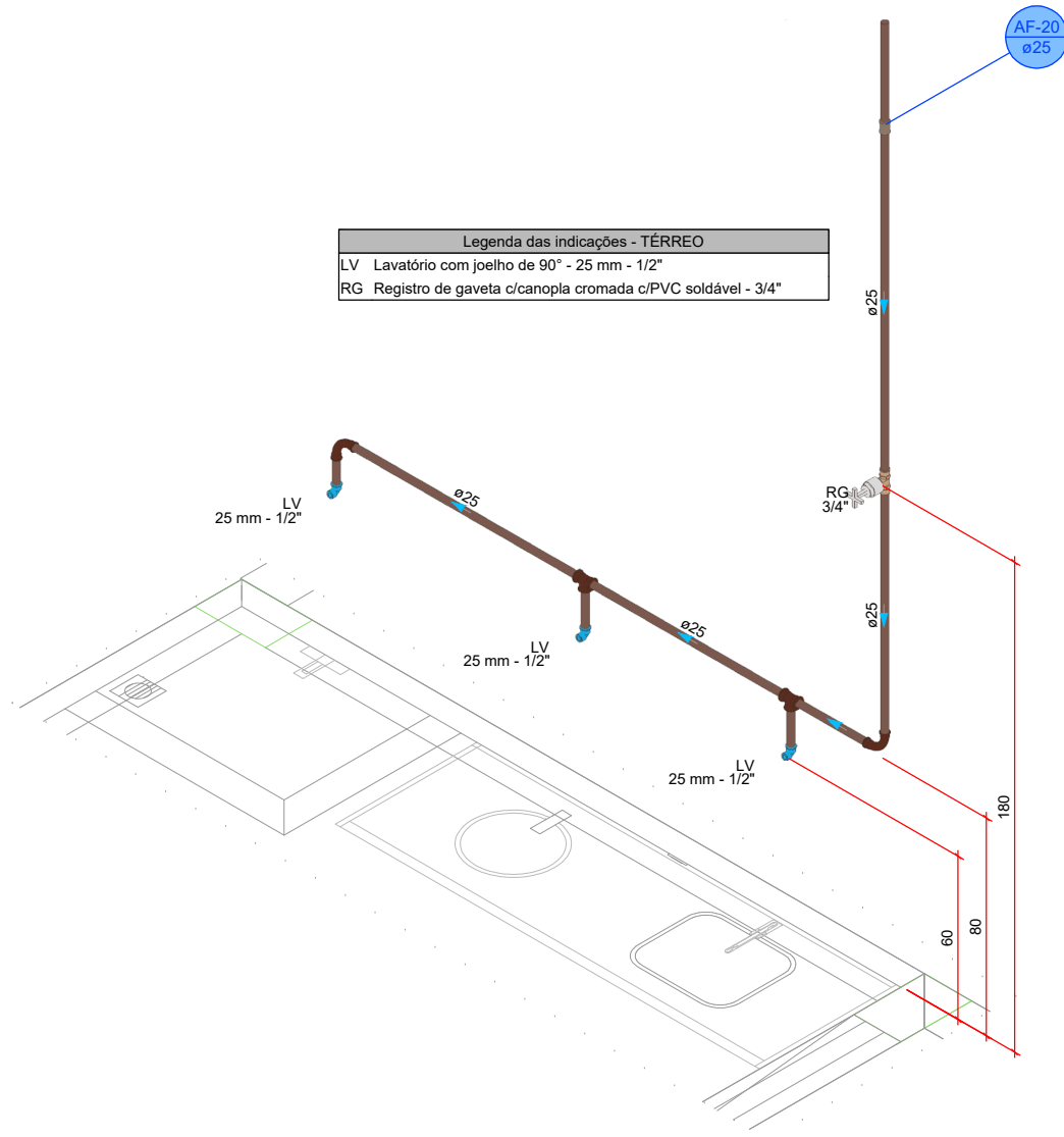
DETALHE HID-15 1:20
