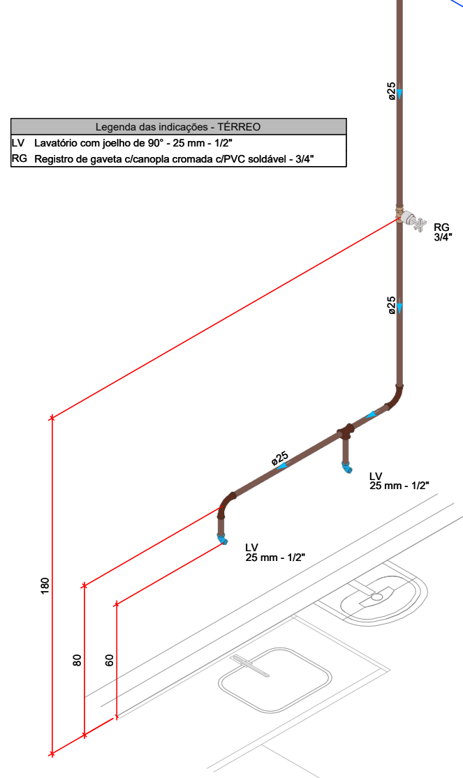
DETALHE HID-19 1:20
