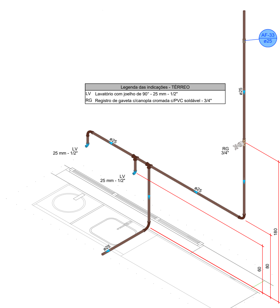
DETALHE HID-28 1:20
