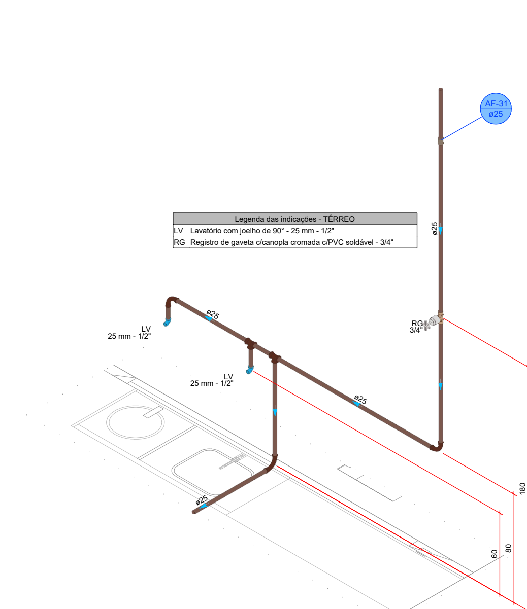
DETALHE HID-26 1:20
