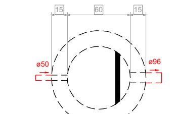
Caixa de gordura - TERREO Planta baixa - ESC. 1:25
