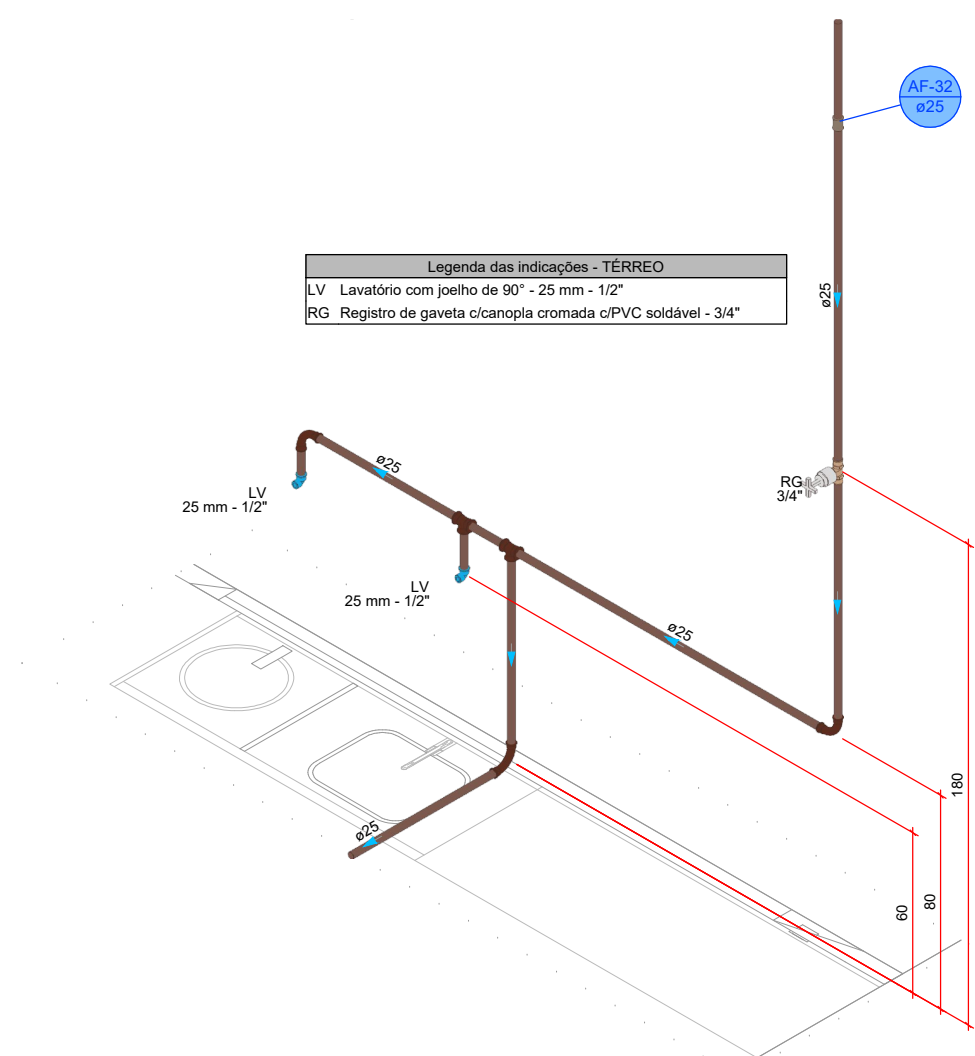
DETALHE HID-27 1:20
