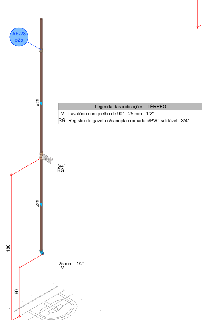
DETALHE HID-29 1:20
