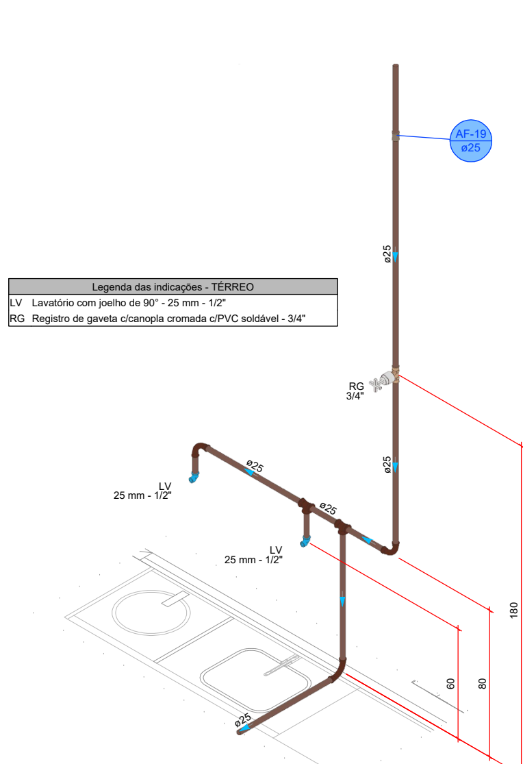
DETALHE HID-18 1:20
