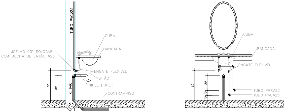
VISTA LATERAL DA LIGAÇÃO DE ÁGUA/ESGOTO Sem Escala VISTA FRONTAL DA LIGAÇÃO DE ÁGUA/ESGOTO Sem Escala
