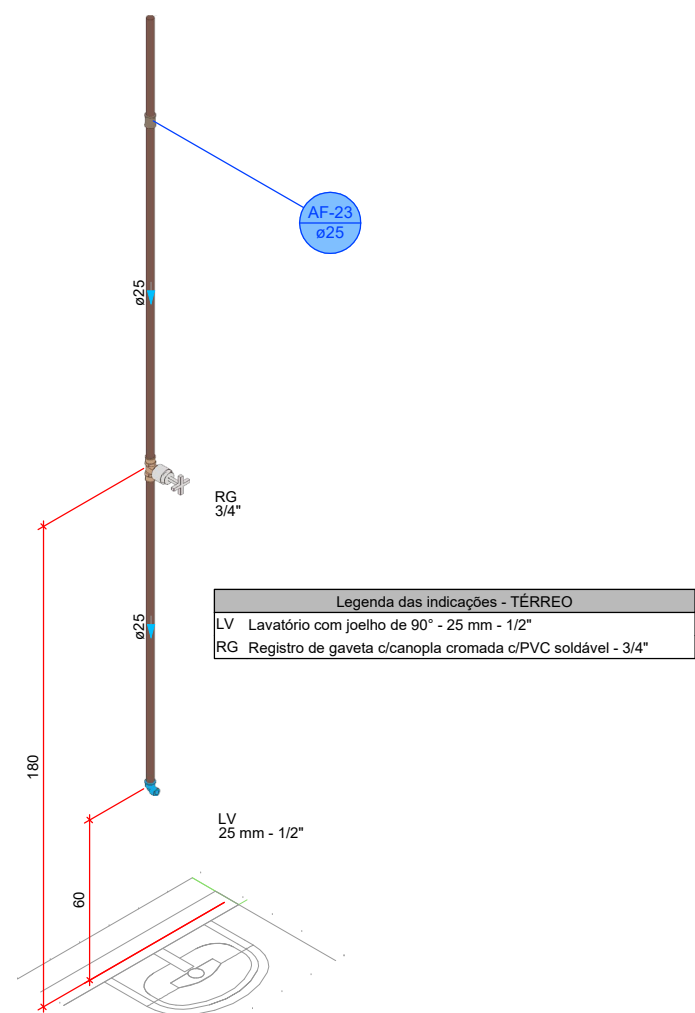
DETALHE HID-21 1:20
