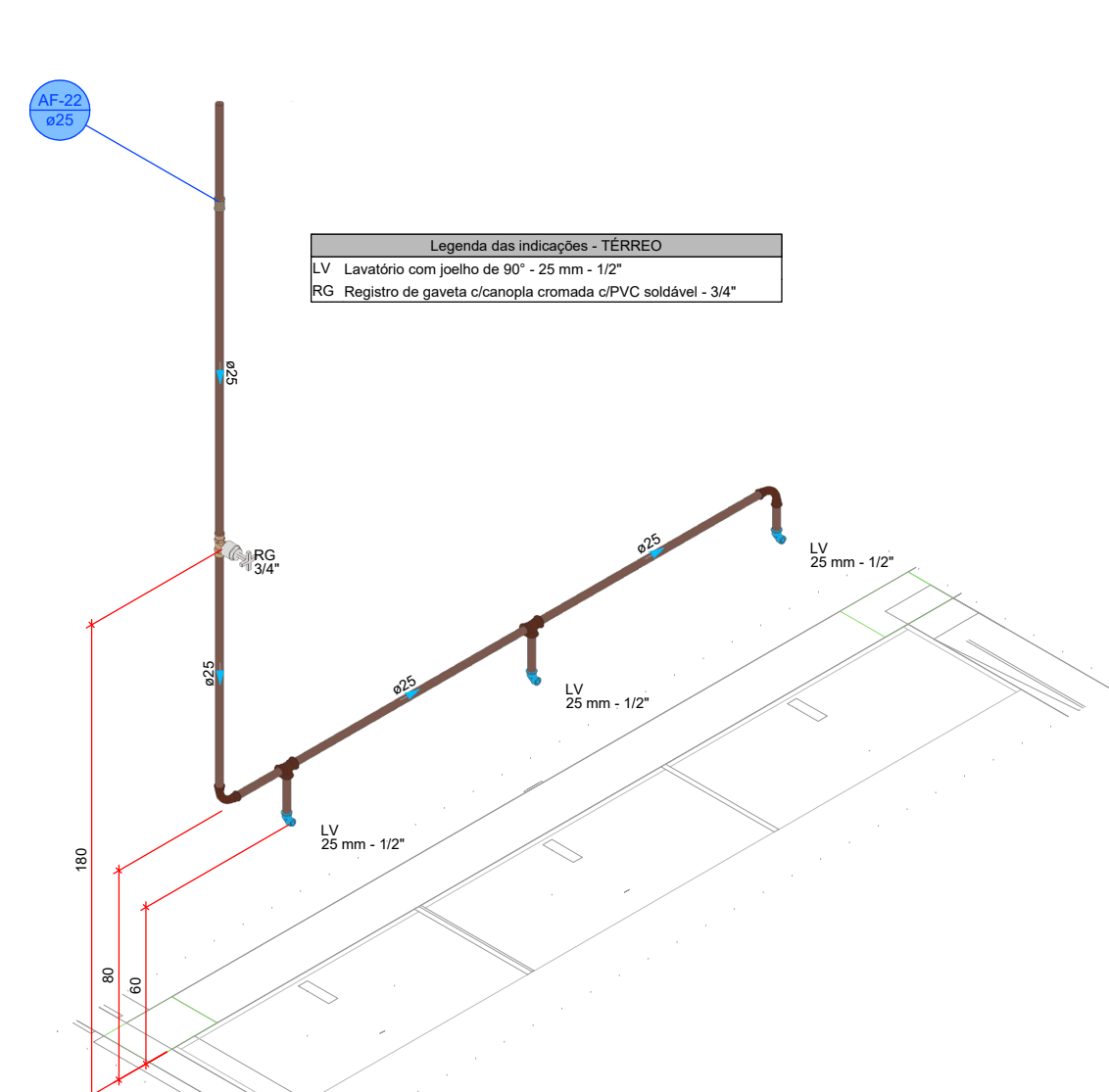
DETALHE HID-20 1:20
