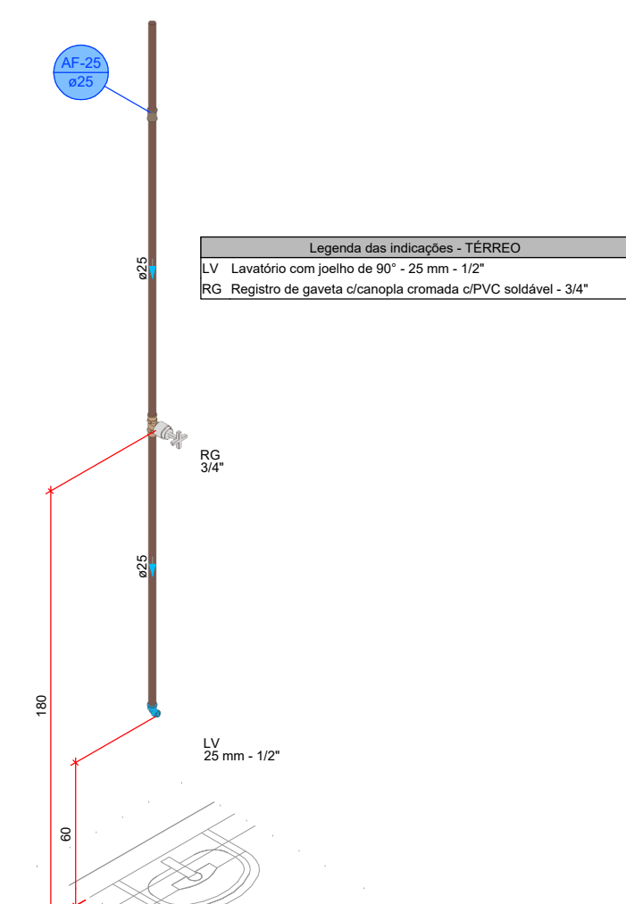
DETALHE HID-24 1:20
