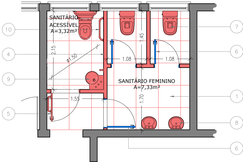
PLANTA BAIXA CONSTRUIR
