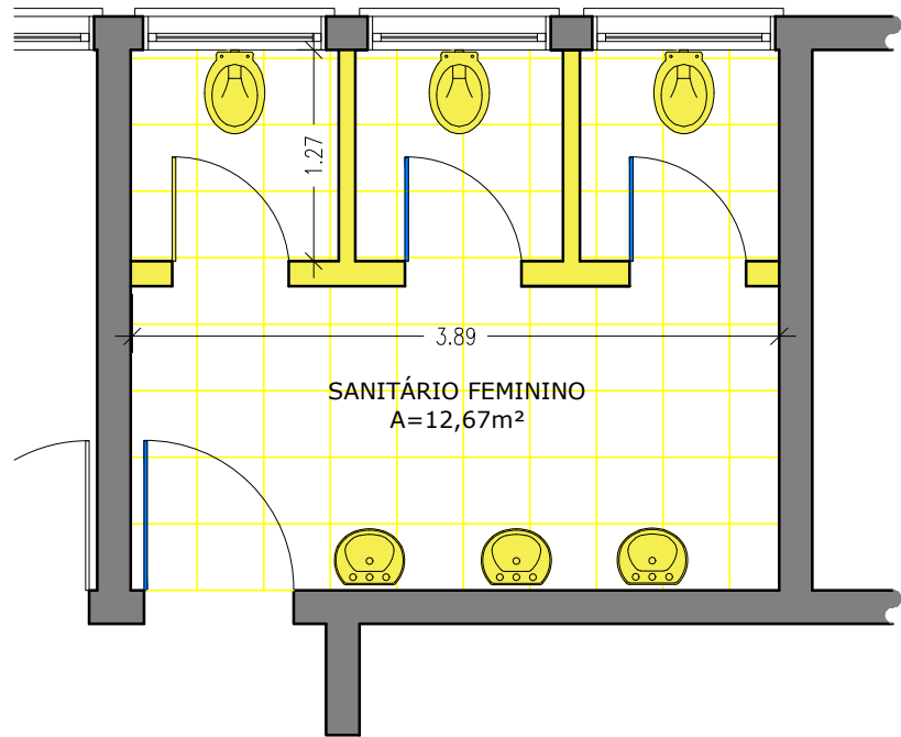
PLANTA BAIXA DEMOLIR
