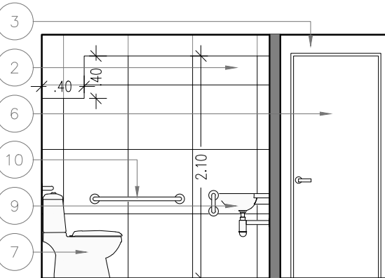
CORTE BB
